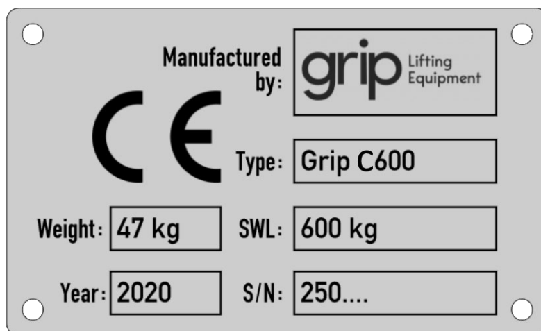
Abbildung 1: Typenschild
