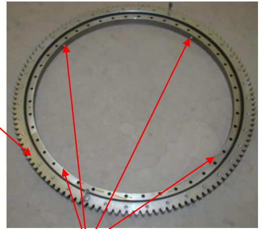
Drehkranz-Laufbahn, Schmierpunkt (11) 4 Schmiernippel
